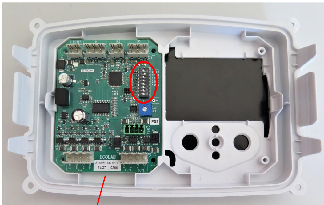
DG1/DG3-DLA PCB mit DIP-Schalter
