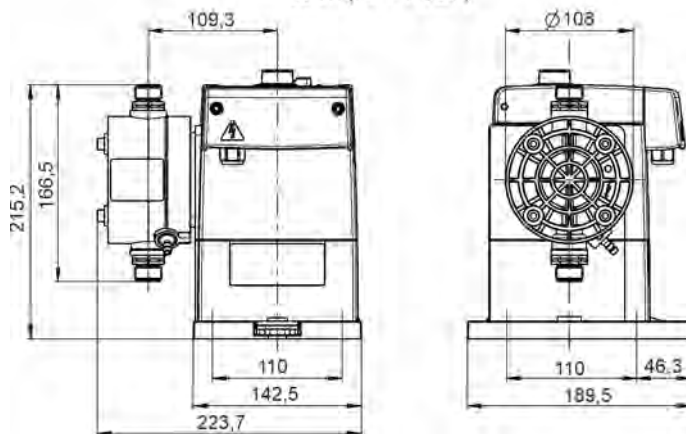
Abb. 36: Abmessungen 30 l/h
