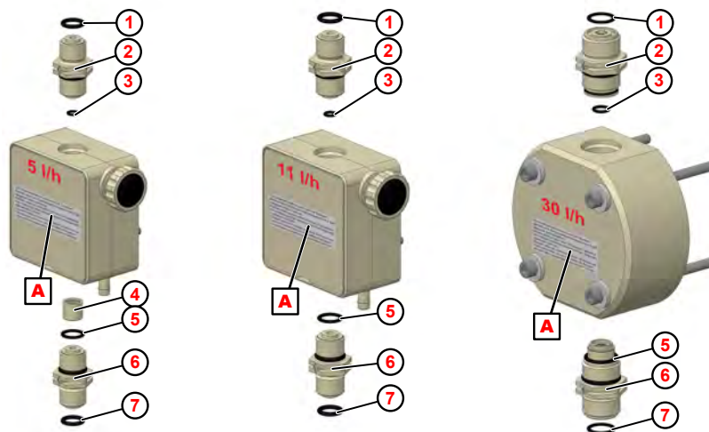
Abb. 20: Austausch von Saug- / Druckventil und Saugventil-Patrone
