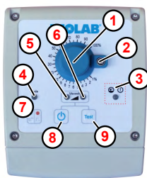
Fig. 13: Élément de commande « EcoUp »
