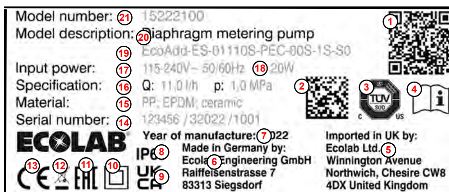
Fig. 34: Plaque signalétique
