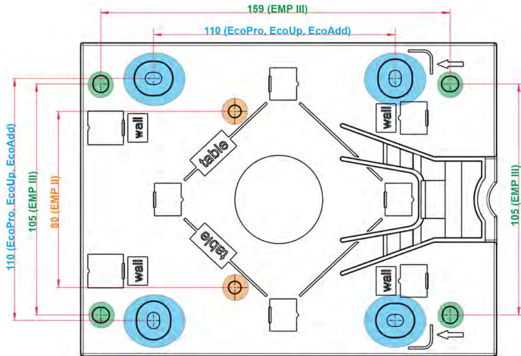
Fig. 37: Dimensiones de la placa de montaje
