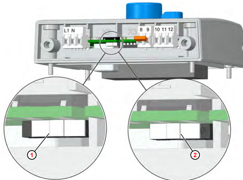
Fig. 14: Attivazione Autostart
