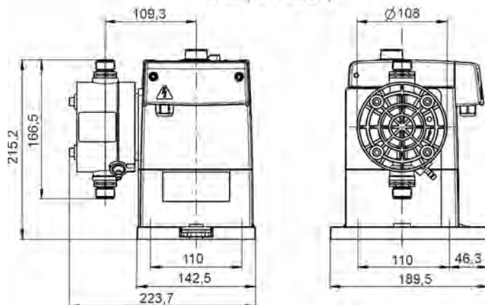
Fig. 36: Dimensiones 5 y 30 l/h
