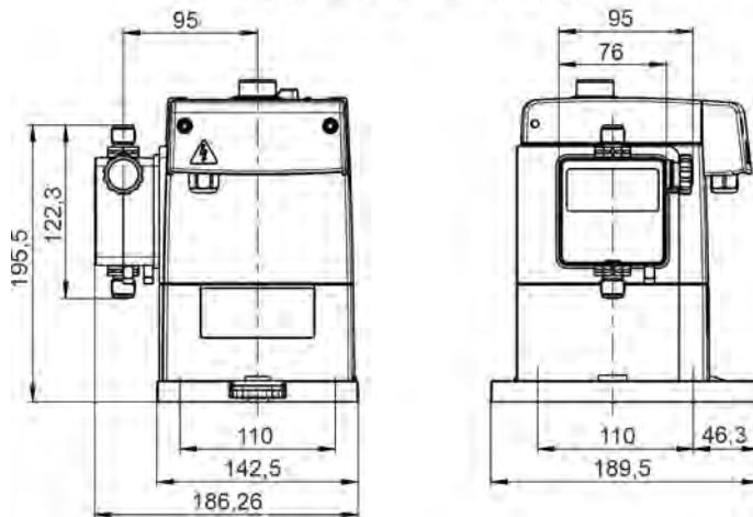
Abb. 35: Abmessungen 5 & 11 l/h
