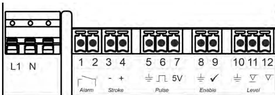
Fig. 12: Configurazione morsetti «EcoUp»
