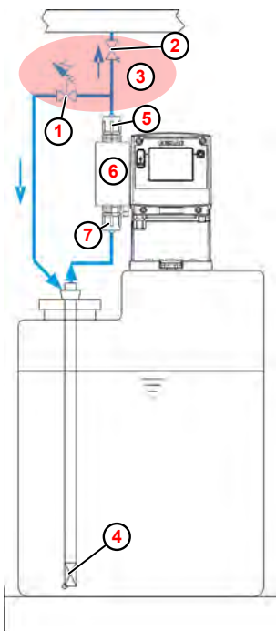
Fig. 6: Esquema de instalación
