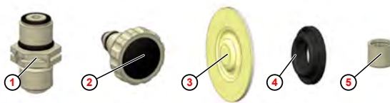
Fig. 25: Set componenti soggetti ad usura
