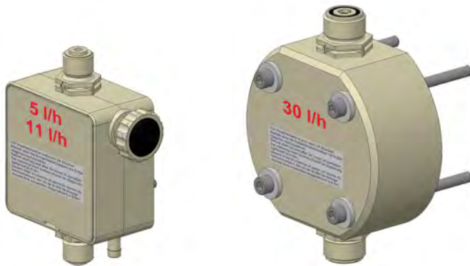
Abb. 2: Pumpenkopfvarianten
