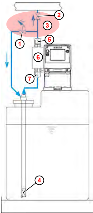
Fig. 6: Schéma de montage
