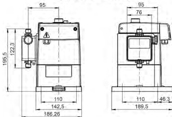
Fig. 35: Dimensioni 5 & 11 l/h
