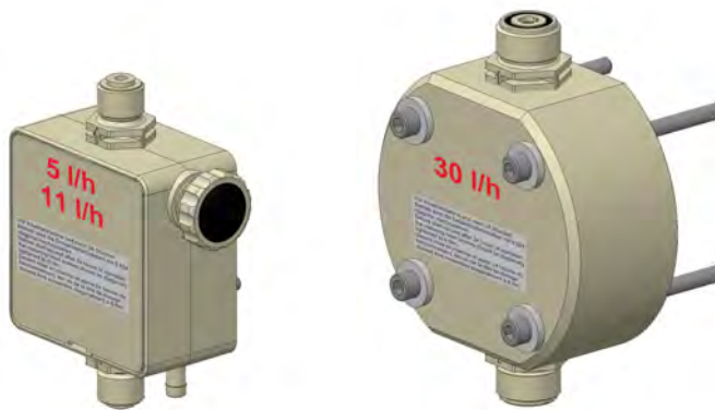
Fig. 2: Variantes de têtes de pompes
