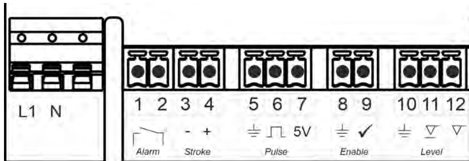
Fig. 12: Affectation des bornes du système « EcoUp »
