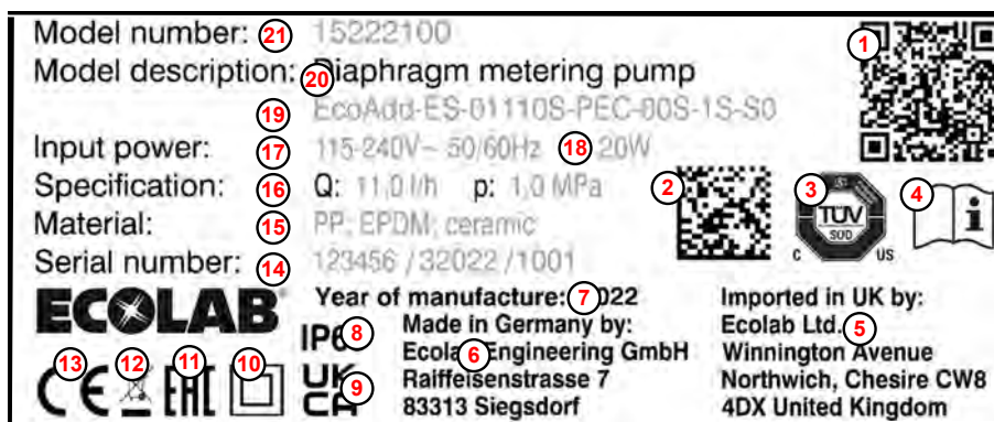
Fig. 34: Placa de características
