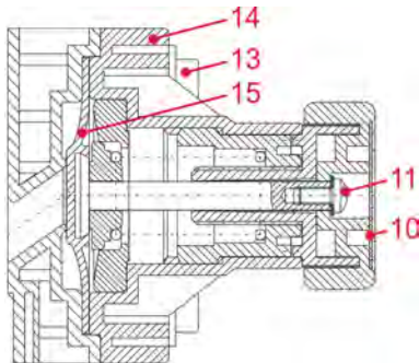
Abb. 6: Austausch der Membrane
