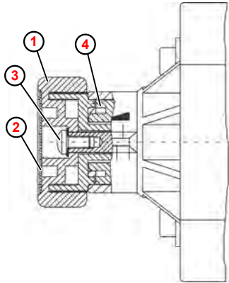
Abb. 4: Einstellen Gegendruck (Druckhaltefunktion)
