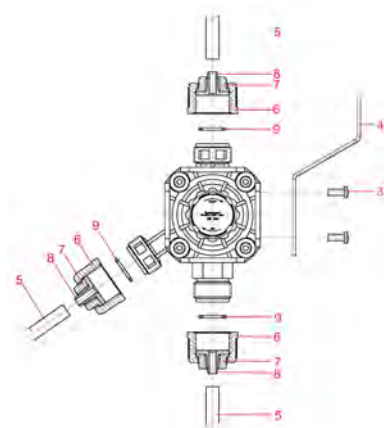
Abb. 2: Installation MFV II-III, Typ 3
