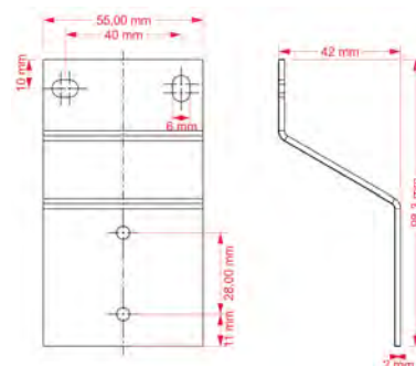
Fig. 8 : Accessoires
