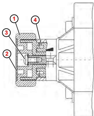
Fig. 4 : Réglage de la contre-pression (fonction de maintien de la pression)
