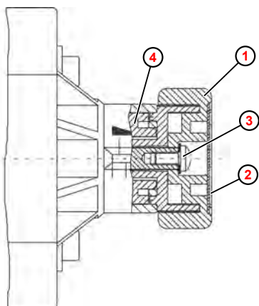
Abb. 5: Einstellen Überdruck (Überdruckfunktion)
