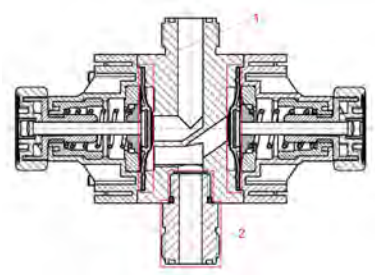
Abb. 7: Ersatzteile
