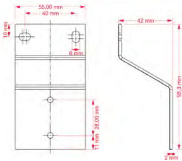
Abb. 8: Zubehör
