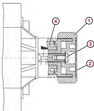
Fig. 5 : Réglage de la surpression (fonction de surpression)
