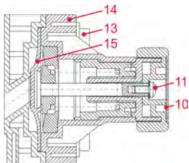
Fig. 6 : Remplacement de la membrane
