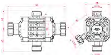
Abb. 9: Abmessungen, Anschlüsse
