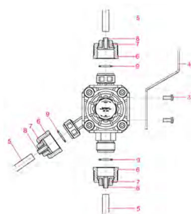
Fig. 2 : Installation de la MFV II-III, type 3
