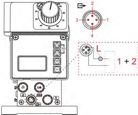
Abb. 7.23 Installation Niveau- bzw. Störmeldeausgang
