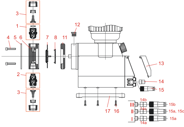
Abb. 13.1 Verschleiß- Ersatzteile (Standard-Ausführung)
