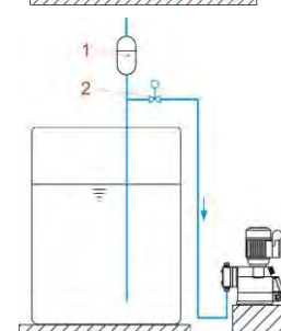
Fig. 7.9 Installation hydraulique : exemples d'installation 9
