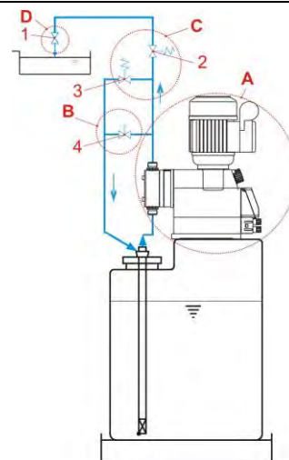
Abb. 7.1 Geräteinstallation Hydraulische Installation Installationsbeispiele 1
