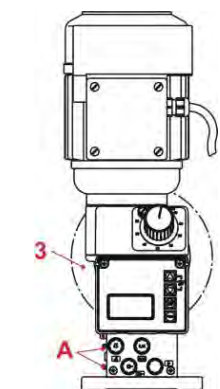
Abb. 5.1 EMP III E60 (vorne)
