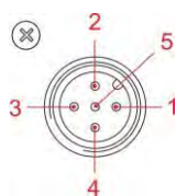
Fig. 8.6 Affectation des connexions – emplacement enfichable VII, (à 5 broches) entrée de l'impulsion de charge et du blocage du dosage
