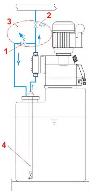
Abb. 6.1 Einbauschema
