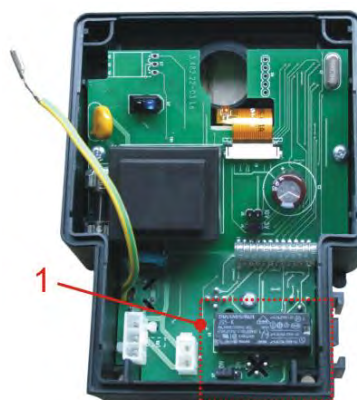
Fig. 7.25 Conversion du matériel pour le contact d'alarme
