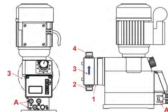
Fig. 5.1 EMP III E60 (front)
