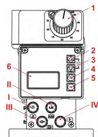
Fig. 5.5 EMP III E60 and EMP III E60 PLUS versions
