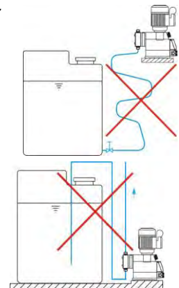
Abb. 7.7 Geräteinstallation: Hydraulische Installation Beispiele 7
