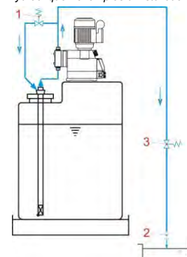
Fig. 7.5 Installation hydraulique : exemples d'installation 5
