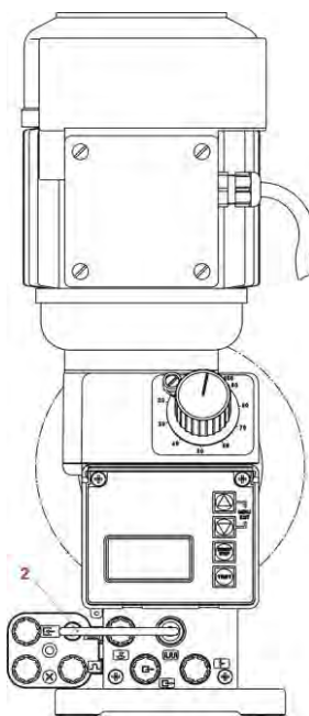
Fig. 8.3 Montage du Dongle-Box 2
