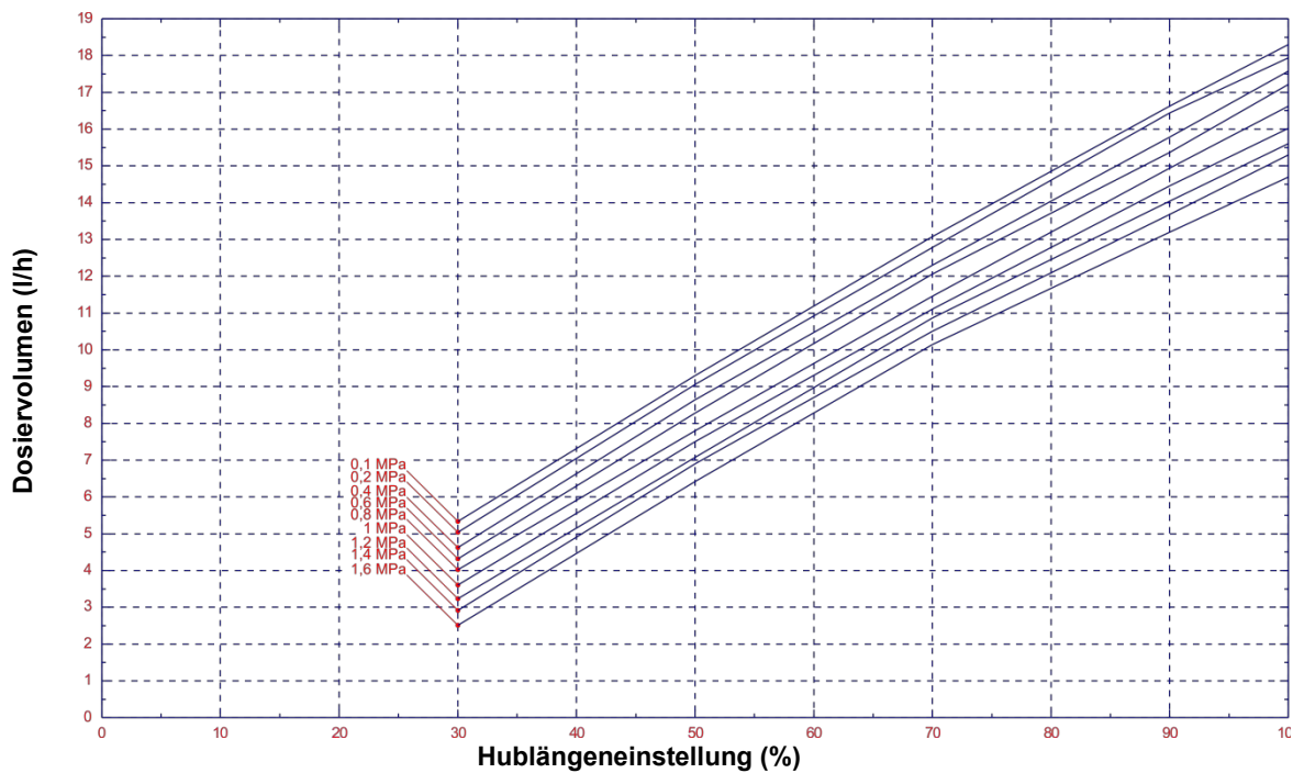
Abb. 14.10 Förderleistung Typ 00160 / 1,6 MPa (16 bar)/ (Sonderversion: höhere Drücke)
