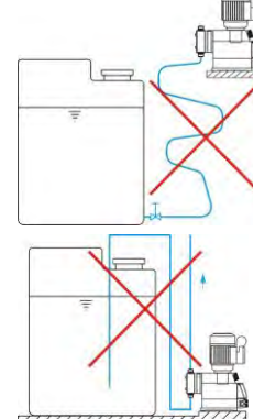
Fig. 7.8 Installation hydraulique : exemples d'installation 8
