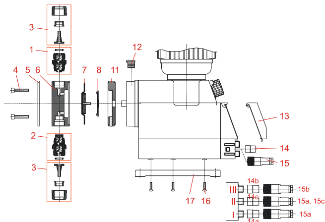
Fig. 13.1 Vue éclatée / Liste des pièces Type 00160, Type 00250, Type 00540
