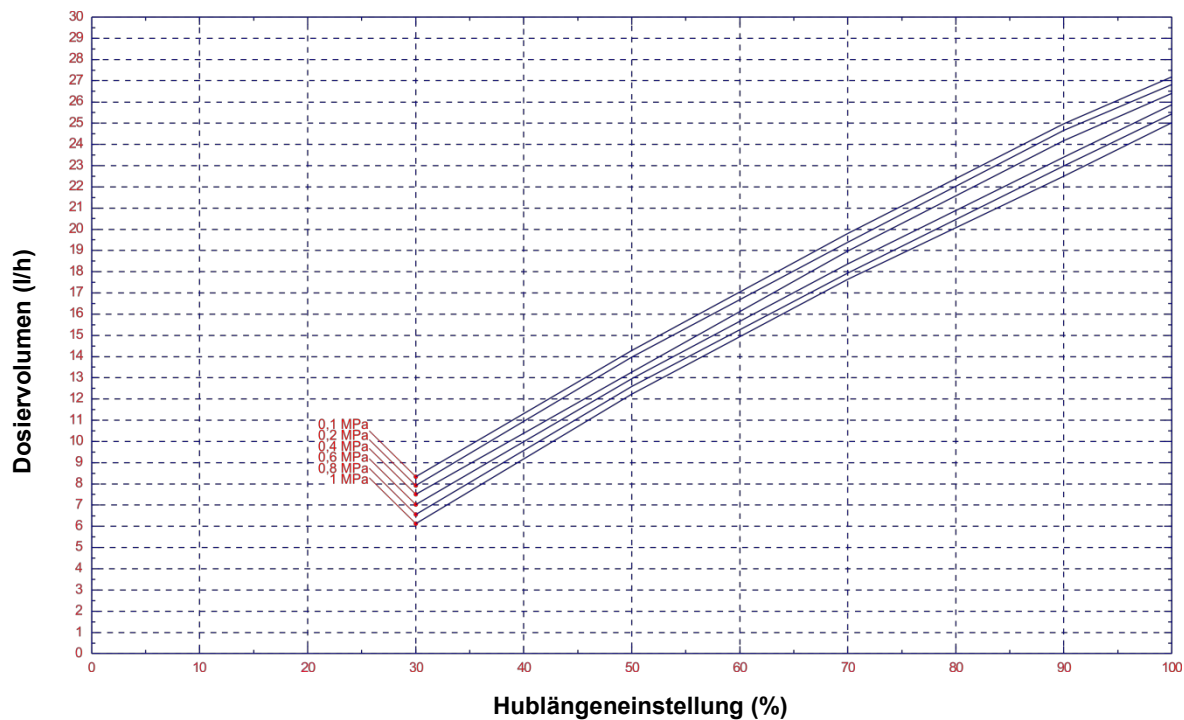
Abb. 14.11 Förderleistung Typ 00250 / 1 MPa (10 bar)
