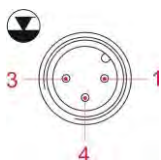
Fig. 7.14 Affectation des - emplacement enfichable I (à 3 broches) entrée du pré-avertissement de niveau et de la signalisation de l'état vide
