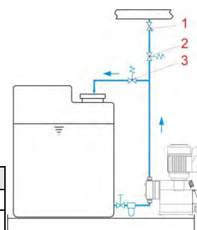
Fig. 7.2 Installation hydraulique : exemples d'installation 2
