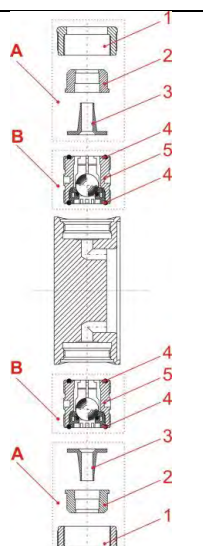
Abb. 11.1 Austausch von Saug- / Druckventil Typ 00800 - 01200
