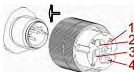
Abb. 14.8 Anschlussstecker / Steuer Ein- und Ausgänge: Pinbelegung / Aderfarben Stecker IV (4-polig)
