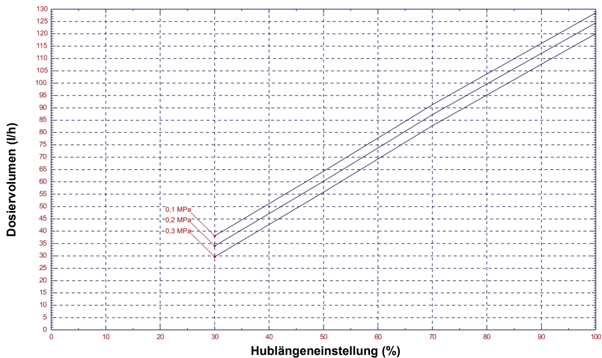
Abb. 14.15 Förderleistung Typ 01200 / 0,3 MPa (3 bar)
