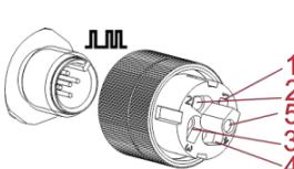
Fig. 14.6 Brochage et couleurs des fils du connecteur II (5-broches)
