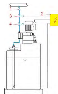
Fig. 7.3 Installation hydraulique : exemples d'installation 3
