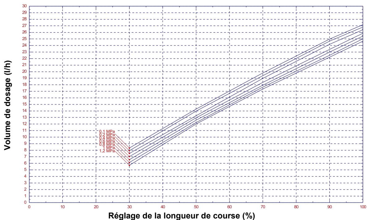
Fig. 14.12 Performance de débit – type 00540 / 1,6 MPa (16 bar) / (version spéciale : pressions plus élevées)
