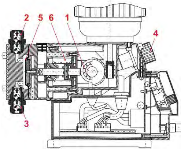
Abb. 4.1 Mechanische Funktionen
