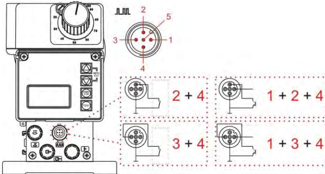
Abb. 7.21 Installation Dosierüberwachung
