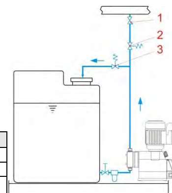
Abb. 7.2 Geräteinstallation: Hydraulische Installation Beispiele 2
