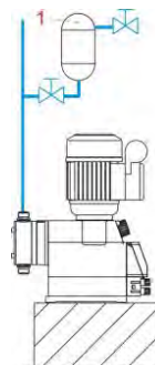
Fig. 7.5 Installation hydraulique : exemples d'installation 5
