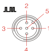
Fig. 14.3 Douille à fiche II
