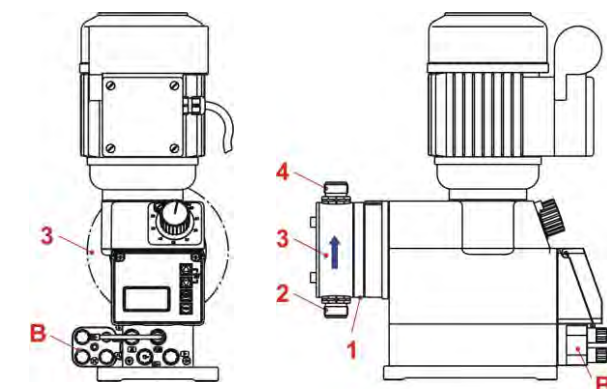
Fig. 5.3 EMP III E60 PLUS (front)
