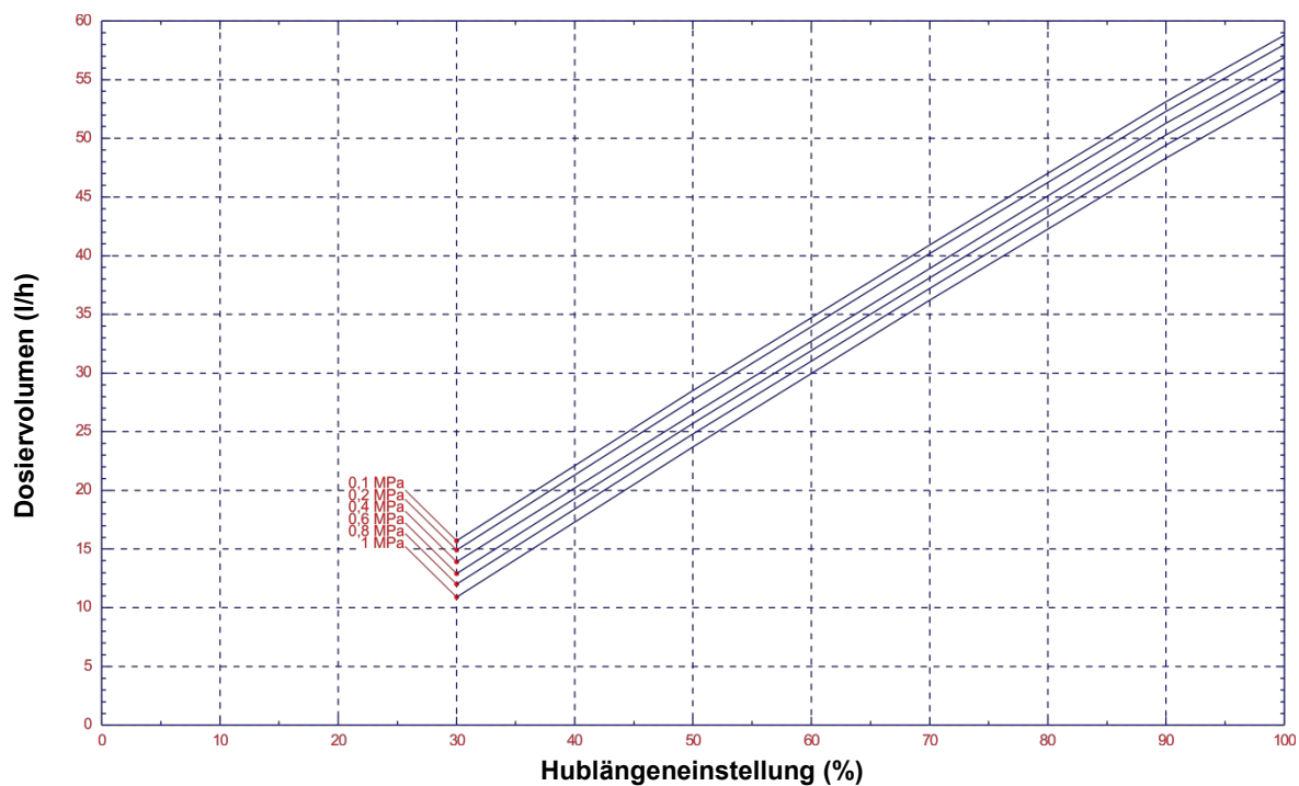
Abb. 14.13 Förderleistung Typ 00540 / 1 MPa (10 bar)
