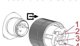
Fig. 14.7 Brochage et couleurs des fils du connecteur III (4-broches)
