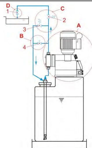
Fig. 7.1 Installation hydraulique exemples d'installation 1
