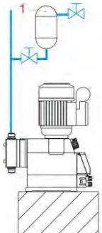
Abb. 7.5 Geräteinstallation Hydraulische Installation Beispiele 5
