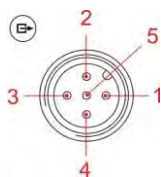
Abb. 8.4 Anschlussbelegung Steckplatz V (5-polig), Dongle-Box
