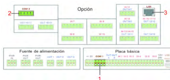
Fig. 1: Anschlussübersicht
