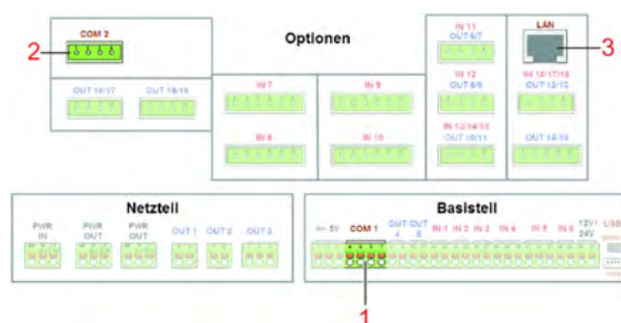
Abb. 1: Anschlussübersicht
