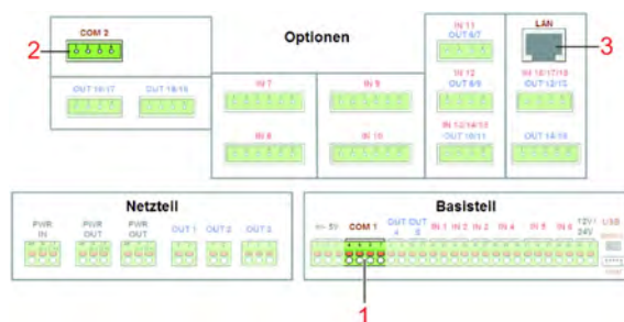
Obr. 1: Přehled připojení
