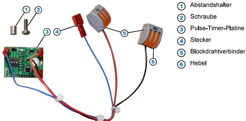
Abb. 1: Timer-Nachrüstset
