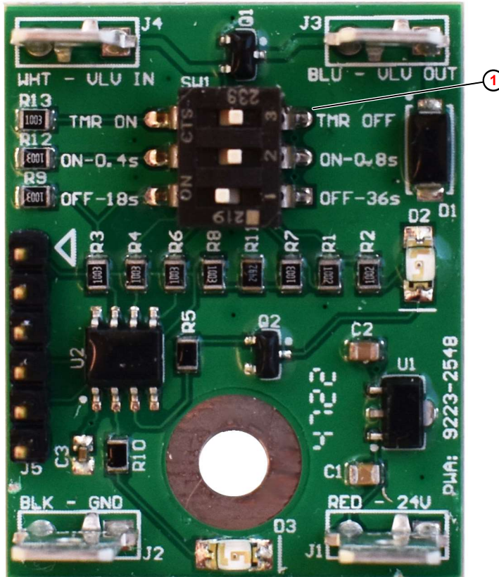
Abb. 4: Deaktivierung des Pulse-Timers
