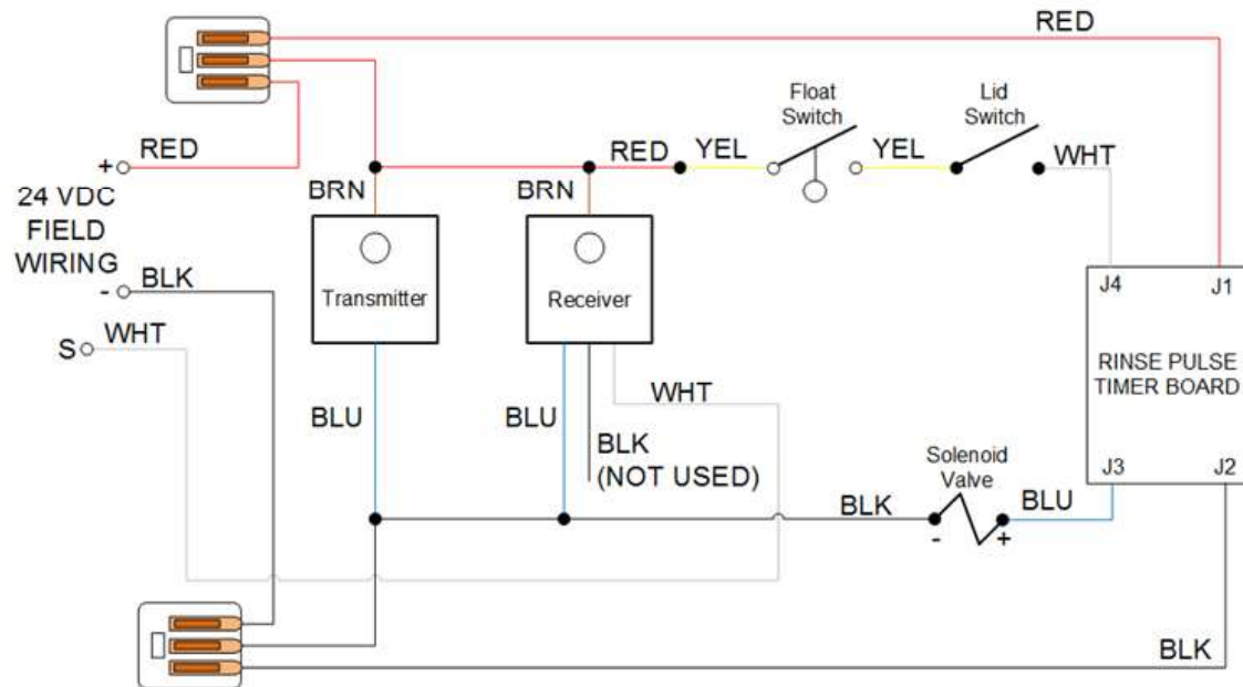
Abb. 2: Verdrahtungsschema APEX Rinse Pulse Timer
