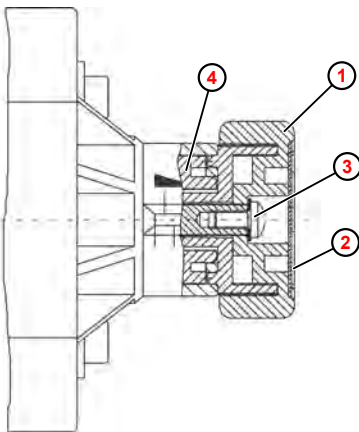
Abb. 5: Einstellen Überdruck (Überdruckfunktion)
