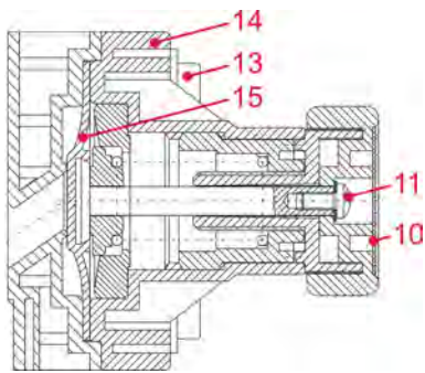
Fig. 7 : Remplacement de la membrane
