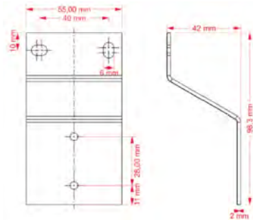
Abb. 9: Zubehör
