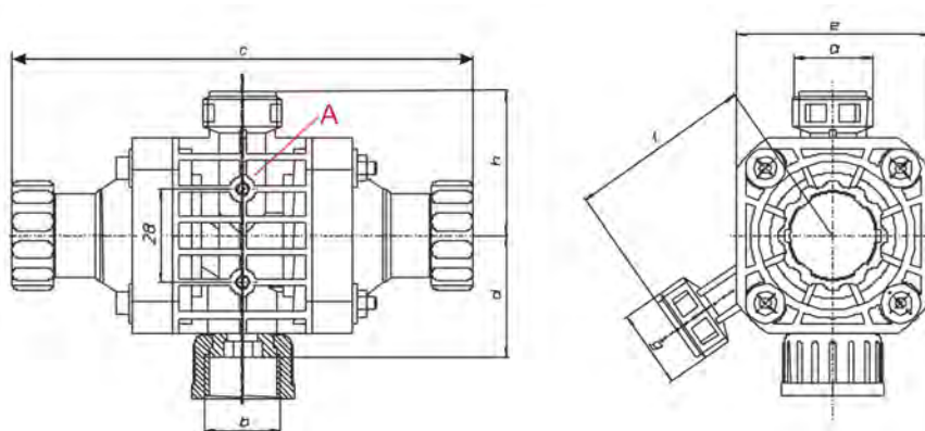
Abb. 10: Abmessungen, Anschlüsse
