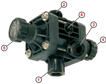
Abb. 1: Aufbau MFV II-III, Typ 1,2
