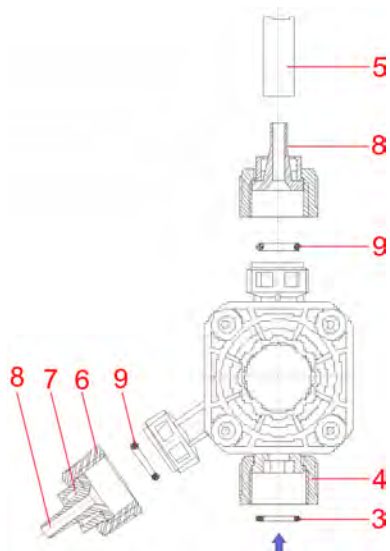
Fig. 2 : Installation de la MFV II-III, type 1, 2
