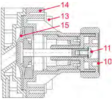
Abb. 7: Austausch der Membrane
