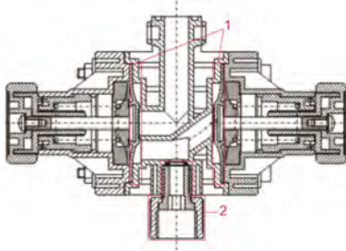
Fig. 8 : Pièces de rechange
