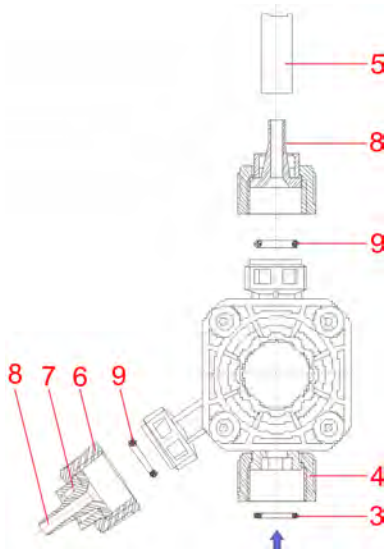
Abb. 2: Installation MFV II-III, Typ 1, 2
