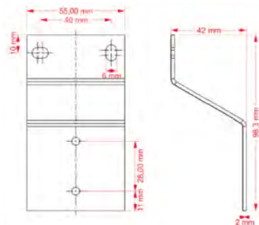
Fig. 9 : Accessoires
