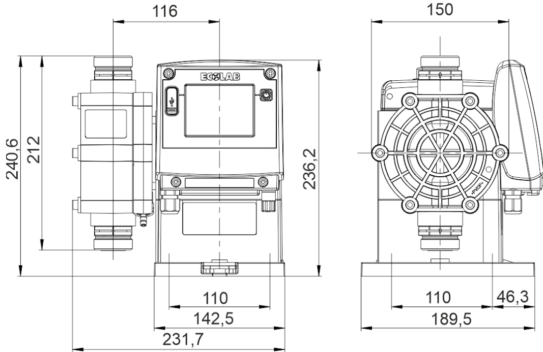
120 l/h (PVDF)
