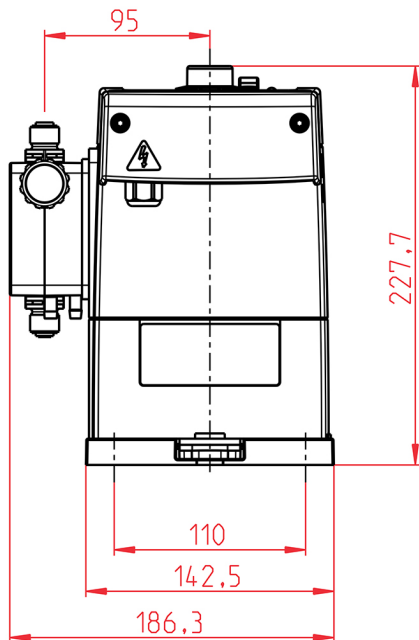
EcoPro/EcoEvo 5 / 10 / 30 l/h
